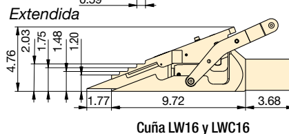
Cuña LW16 y LWC16
