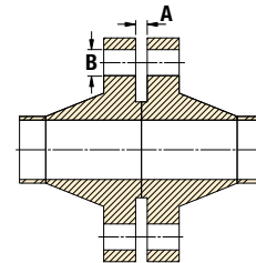
Dimensiones de brida
