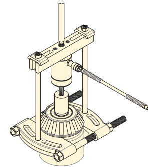
▲ Extractor de cruceta con cojinete Separador en una aplicación
