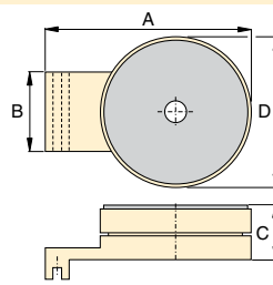
Placa de nivelación ES60, ES80
