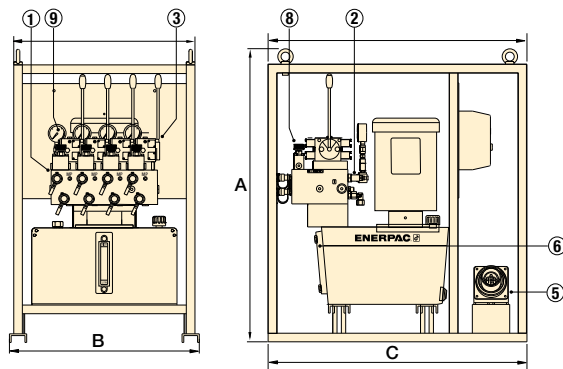
◀ Serie SFP con ta (se muestra con 4 salidas de flujo dividido)
