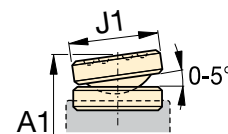
Silleta de inclinación serie CATS
