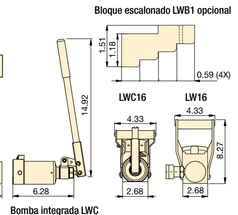
Bloque escalonado LWB1 opcional
