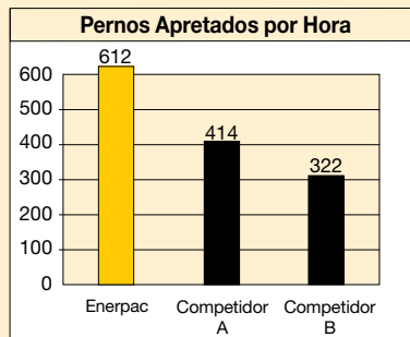
Pruebas de laboratorio internas en un procedimiento de apriete estándar de la brida de una tubería con 14 pernos de 1 7/8".
