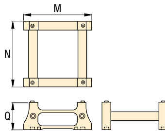
Bloque de soporte temporal
