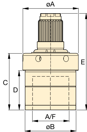
STTLS para ajuste de estría de la serie S
